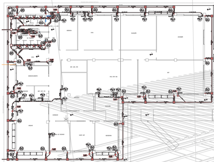
PROJETO HIDROSSANITÁRIO
