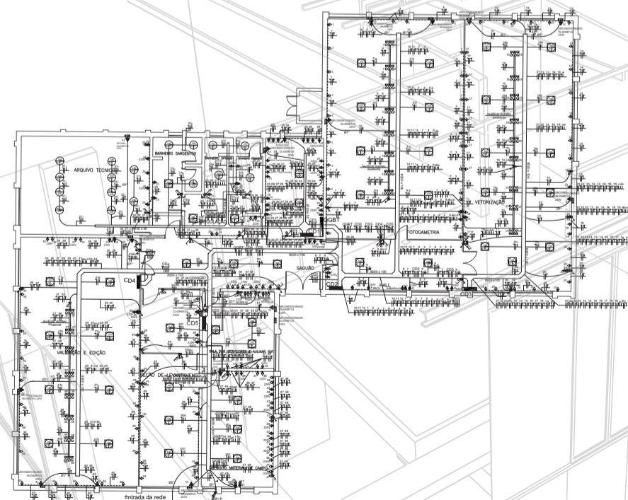
PROJETO ELÉTRICO
